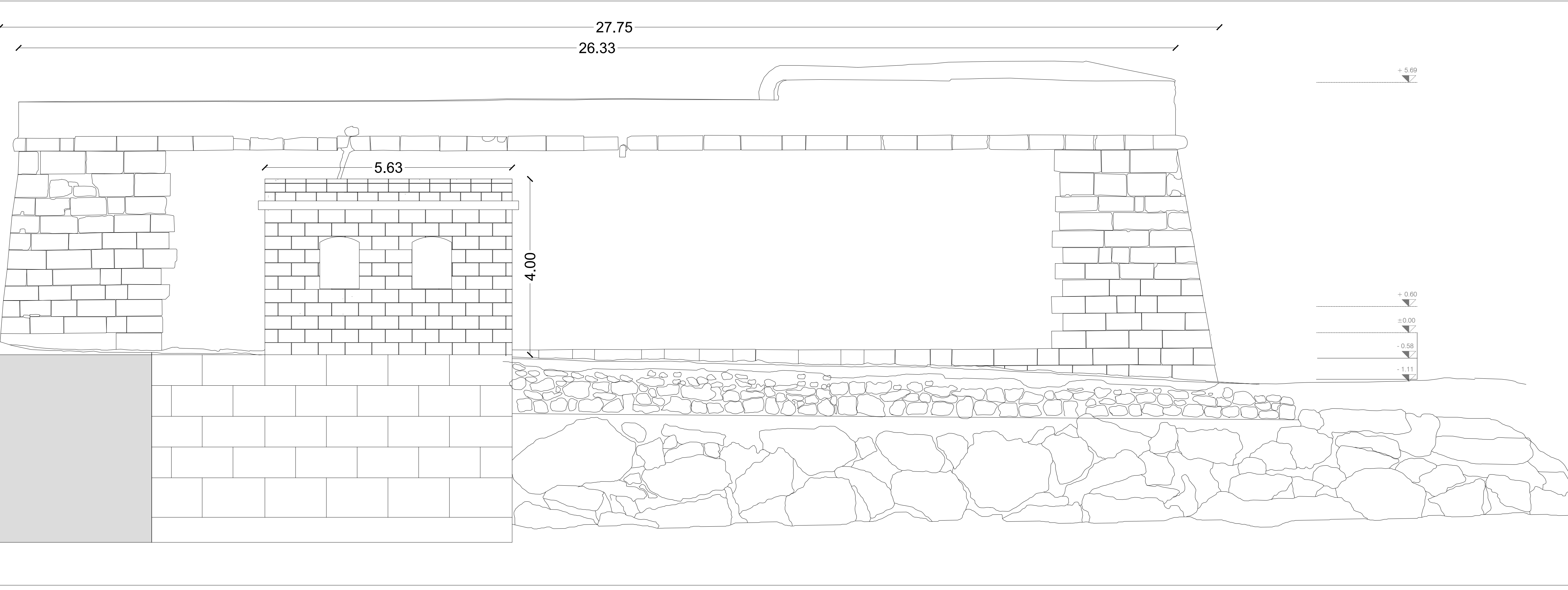
PROSPETTO Stato di fatto - Scala 1:50
